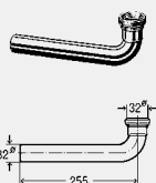
Отводящее колено 90° - хромированная латунь Модель 5622.2
